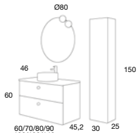
CARMEN 80 cm | 2 Cajones | Color 18 Tirador Rondo Negro Mueble + Encimera K-Negro + Lavabo Circulo K-Negro
